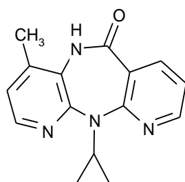
Nevirapine
