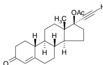
Norethisterone Acetate CAS : 51-98-9
